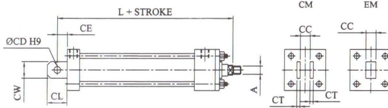
CAP END CLEVIS (CM/EM)
